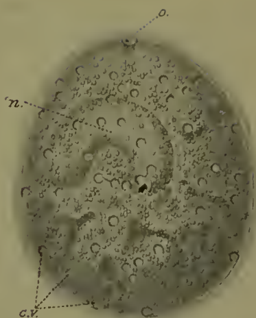
Fig. 83. Ichthyophthirius multifiliis (nach Bütschli).
